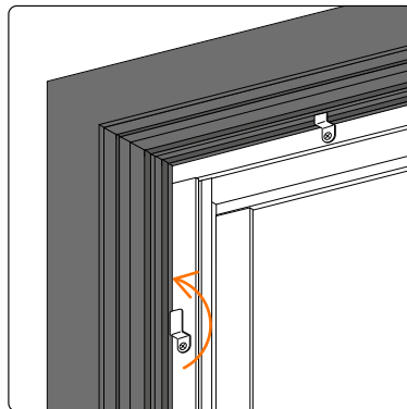
Positionnez les crochets de fixation
