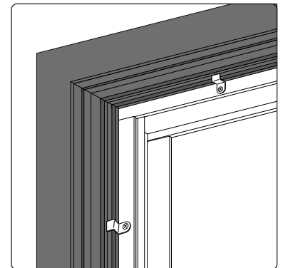
Tournez pour fixer au profil
